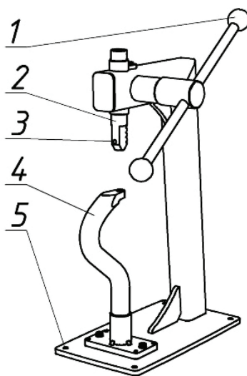
Рис. 5. Станок для клепки коньков
