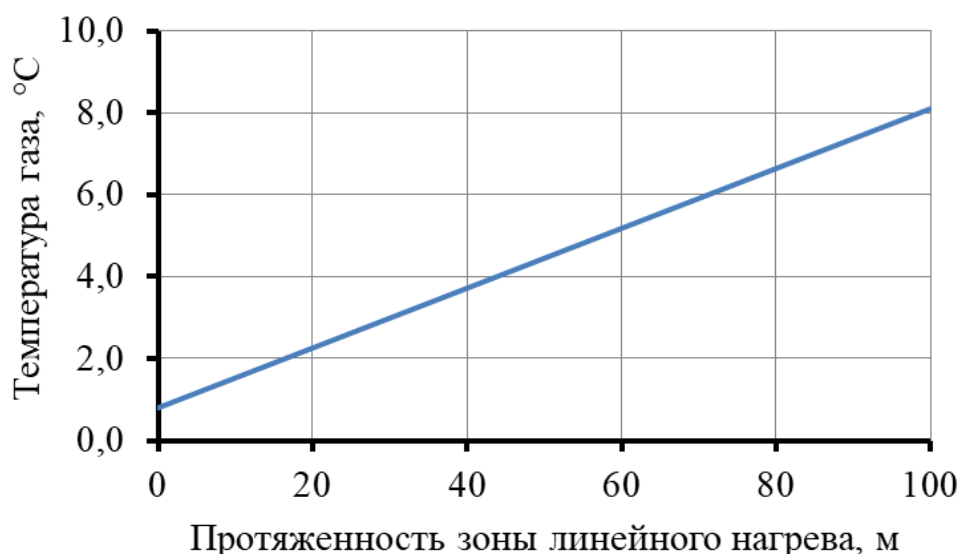
Рис. 1. Нагрев газа на участке путевого подогрева при температуре стенки трубы 40 °С (рабочее давление 0,3 МПа, расход 0,036 млн. м³/сут.)
