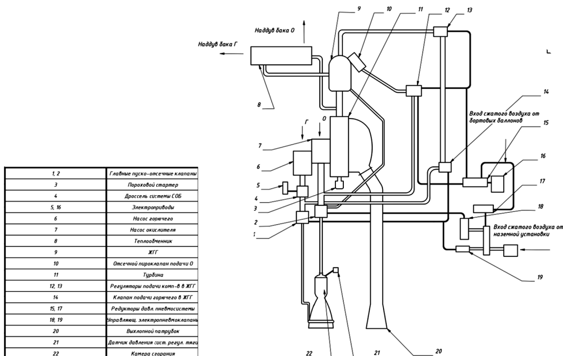
Рис. 4. Пневмогидравлическая схема ЖРД [7]
