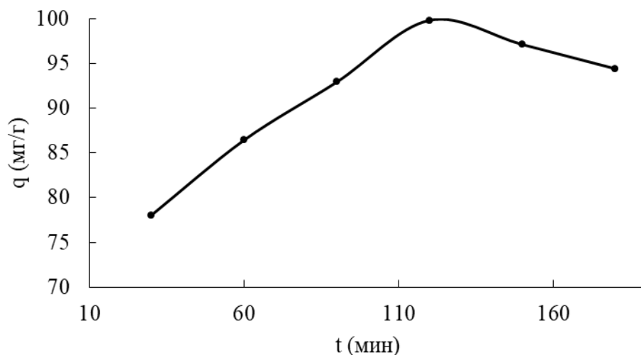
Рис. 2. Влияние времени на адсорбционную емкость скорлупы арахиса с \text{Fe}_3\text{O}_4 для метиленового синего
