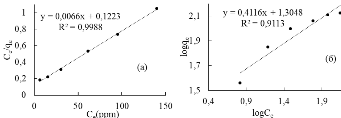
Рис. 5. Изотермы адсорбции Ленгмюра (а) и Френдлиха (б) скорлупы арахиса с \text{Fe}_3\text{O}_4 для метиленового синего
