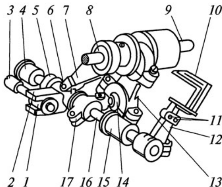
Рис. 1. Механизм петлителей швейных машин Зингер на базе машины 876 кл.
