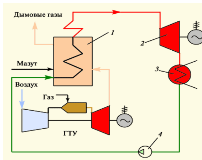
Рис. 2. Схема сбросной парогазовой установки
