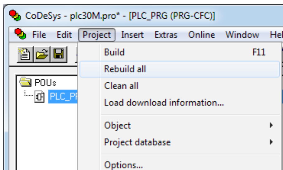
Рис. 8. Проект/Компилировать все
