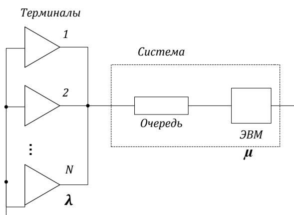
Рис. 1. Структура модели
