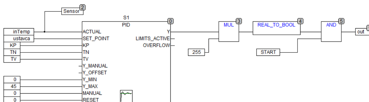
Рис. 14. ПИД регулятор на языке CFC
