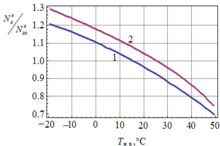
Рис. 1. Зависимость электрической мощности ГТУ от температуры наружного воздуха при номинальной нагрузке (1) и пиковой нагрузке (2). N_z^э , N_{z0}^э — текущая электрическая мощность и мощность базового режима (при +15 °C)
