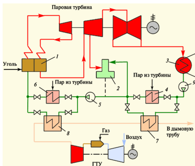
Рис. 3. Принципиальная схема парогазовой установки с вытеснением регенерации
