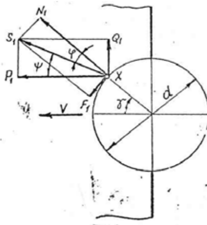
Рис 1. Силевая схема взаимодействия микрозубца с полуфабрикатом (в горизонтальной плоскости)
