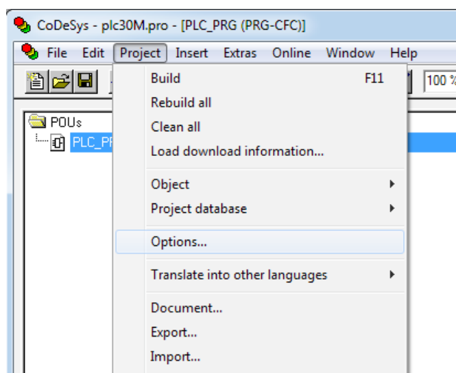
Рис. 5. Проект/Опции
