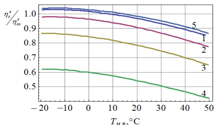
Рис. 2. Зависимость электрического КПД ГТУ от температуры наружного воздуха при разной нагрузке: номинальная (1), 75% (2), 50% (3), 25% (4) и пиковая (5). \eta_z^э , \eta_{z0}^э — значения КПД в текущем режиме и базовом режиме соответственно
