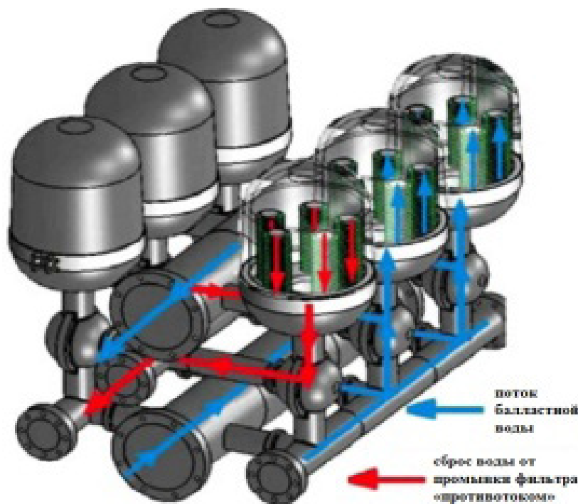
Рис. 2. Схема фильтра очистки балластной воды
