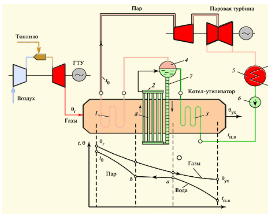
Рис. 1. Принципиальная схема простейшей парогазовой установки утилизационного типа
